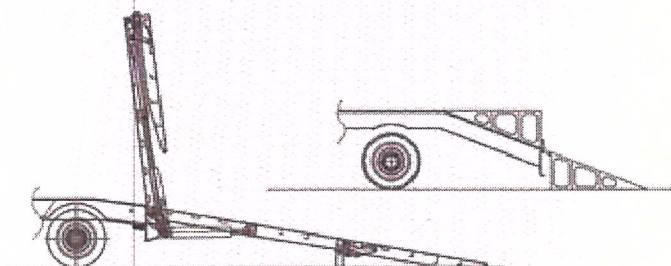
Варианты исполнения трапов
