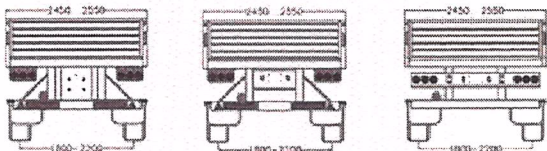
вид сзади для LXP9400LB2
