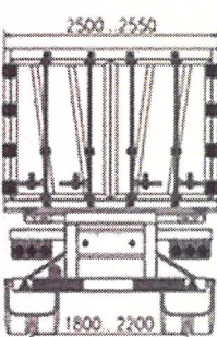
вид сзади для LXP9400XXYZ2
