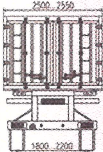
вид сзади для LXP9400XXYZ2D
