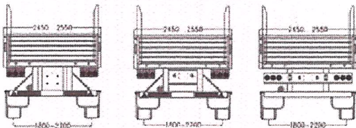
вид сзади для LXP9400LB2
