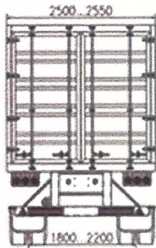
вид сзади для LXP9400XXY2
