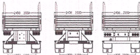
вид сзади для LXP9400LB2
