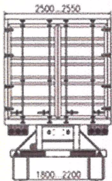
вид сзади для LXP9400XXY2D
