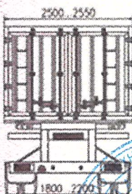
вид сзади для LXP9400XXYZ2
