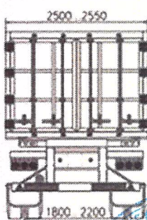
вид сзади для LXP9400XXYZ2
